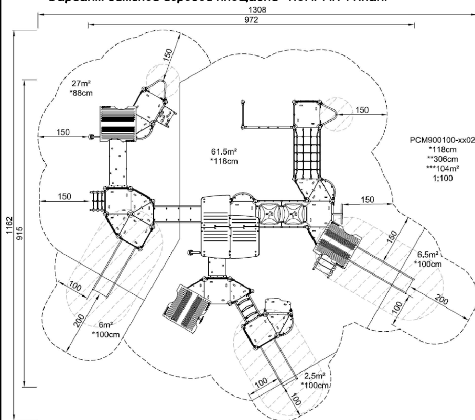
Вариант детской игровой площадки "КОМПАН". План.
